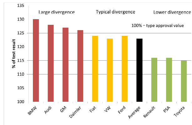
Diag. 1: Razkorak med uradnimi rezultati testiranj in povprečnimi rezultati doseženimi med vožnjo v l. 2011 (ICCT, 2013)
